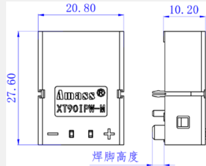
焊脚高度
