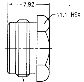
CLAMP NUT
