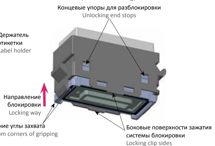
Модуль типа 1767 PA в заблокированном виде (для установки на планку) Locked 1767 PA module (for rail mounting)
