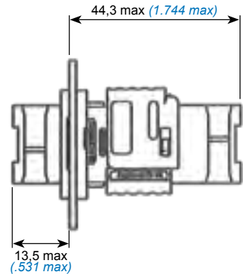
Fiche longue / Embase collerette longue Long plug / Long flanged receptacle
