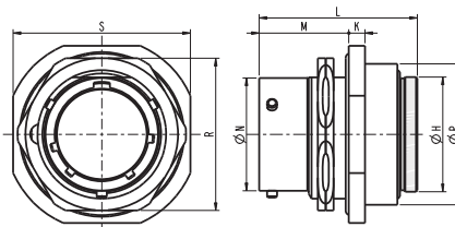
Jam nut receptacle with grommet backnut. Embase à fixation par écrou avec écrou serre-fils.
