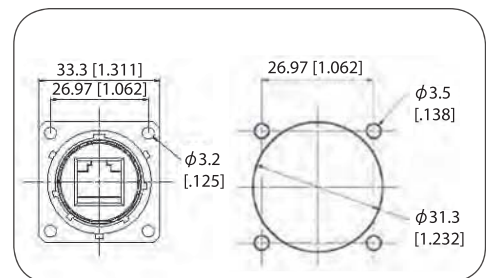
Panel Drilling Découpe de Panneau
