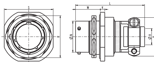
Jam nut receptacle with cable clamp backshell. Embase à fixation par écrou avec raccord serre-câble.
