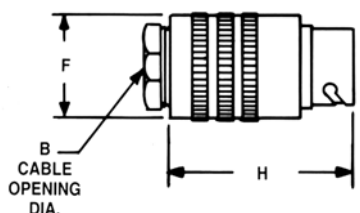
Cable Receptacle
