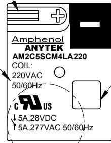
A(当负载为5A 印字图)
