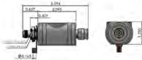
• LP-GPX-05-TFM 1000 - 2000MHz TNC Type F/M
