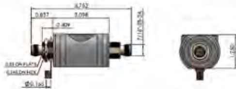
• LP-GPX-05-TFF 1000 - 2000MHz TNC Type F/F
