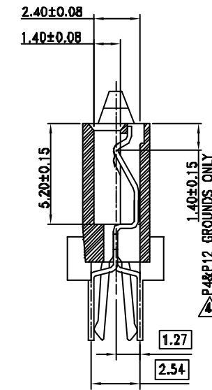
SECTION N-N 2:1
