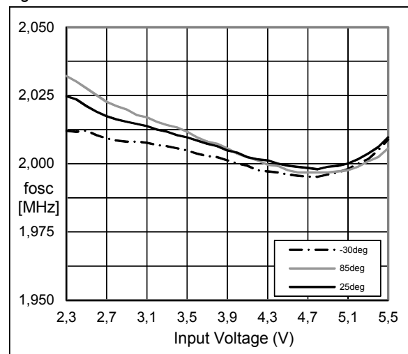
Figure 14. fosc vs. VIN
