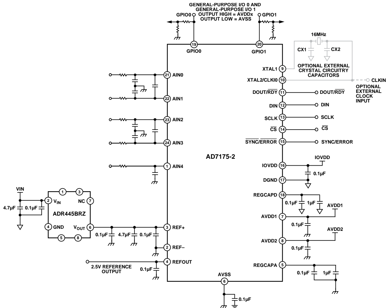
图44. 典型连接图
