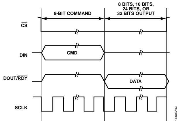
图47. 读取一个寄存器 (8位命令和寄存器地址，随后是8位、16位或24位数据；DOUT上的数据长度取决于所选的寄存器)
