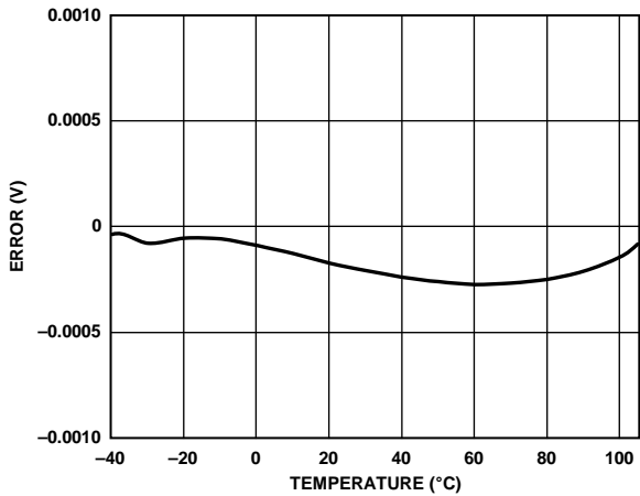
图31. 基准电压绝对误差与温度的关系
