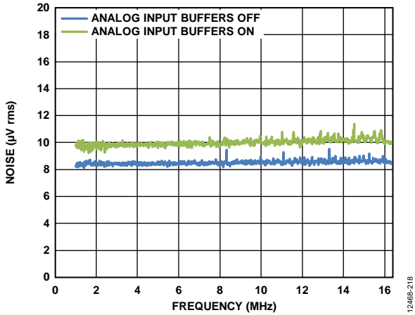
图18. 噪声与外部主时钟频率的关系，模拟输入缓冲器开启和关闭
