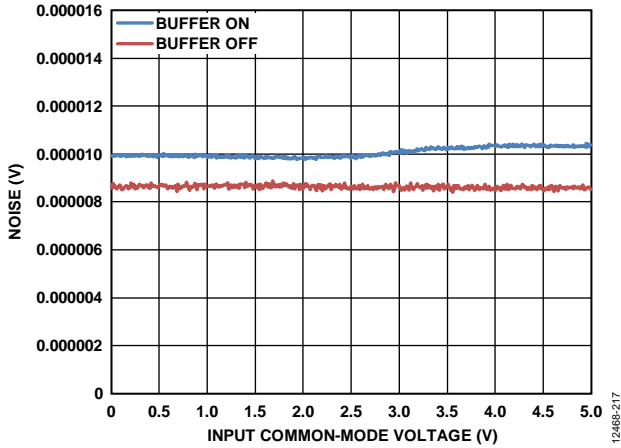
图17. 噪声与输入共模电压的关系，模拟输入缓冲器开启和关闭
