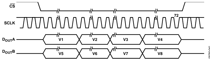
图44.采用双 D_{OUT} 线路的AD7609串行接口
