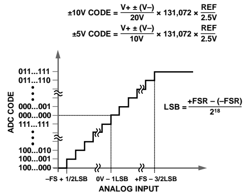
图37. AD7609传递特性
