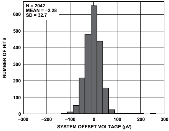
图7. 典型系统失调电压分布图
