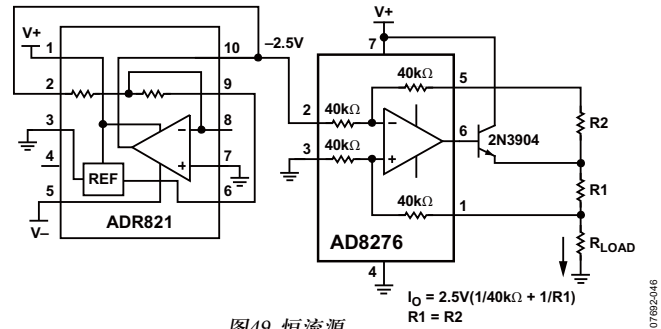
图49. 恒流源
