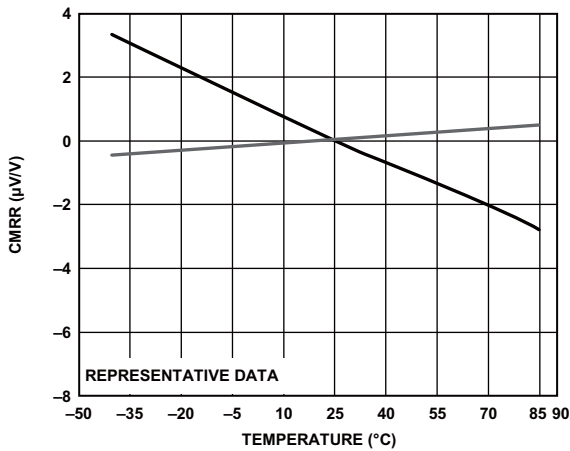
图9. CMRR与温度的关系, 归一化至25°C
