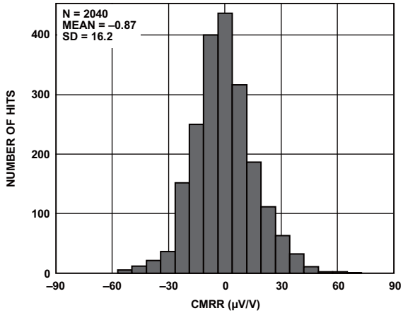
图8. 典型共模抑制分布图
