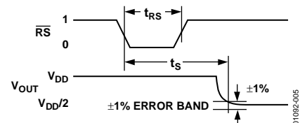
图5. 复位时序图
