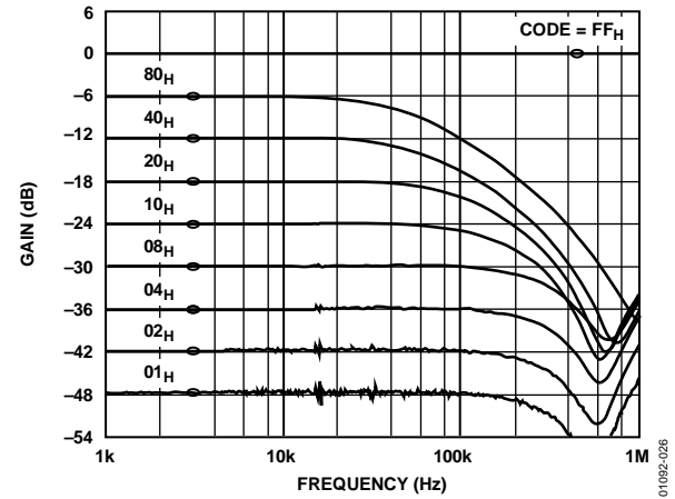
图26. 100 kΩ增益、频率与代码的关系
