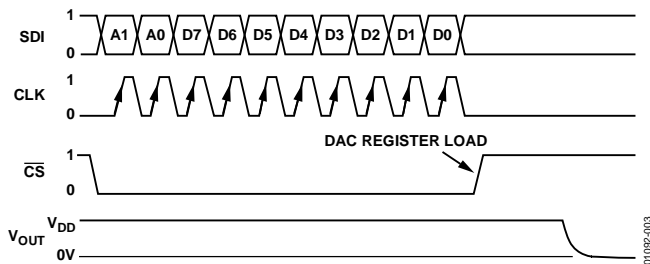
图3. 时序图
