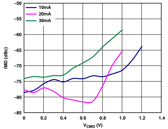
图72. IMD与输出共模电压的关系 ( f_{OUT} = 161 \text{ MHz} , R_{LOAD} = 50 \Omega 差分, I_{FS} = 10 \text{ mA} , 20 \text{ mA} 和 30 \text{ mA} )
