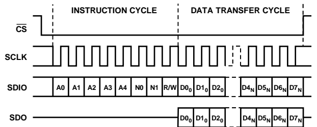
图40. 串行寄存器接口时序(LSB优先)
