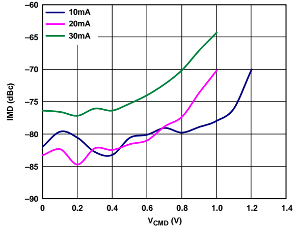
图71. IMD与输出共模电压的关系 ( f_{OUT} = 61 \text{ MHz} , R_{LOAD} = 50 \Omega 差分, I_{FS} = 10 \text{ mA} , 20 \text{ mA} 和 30 \text{ mA} )
