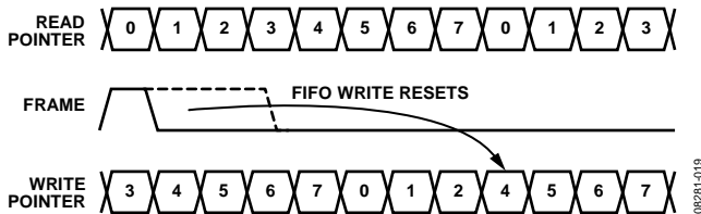
图47. FRAME输入与写指针值的关系(数据速率模式)
