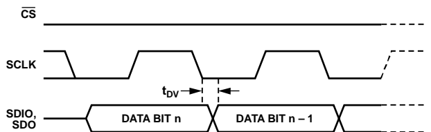
图42. 串行端口寄存器读操作时序图
