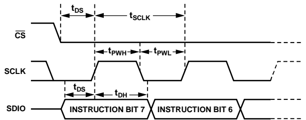
图41. 串行端口寄存器写操作时序图
