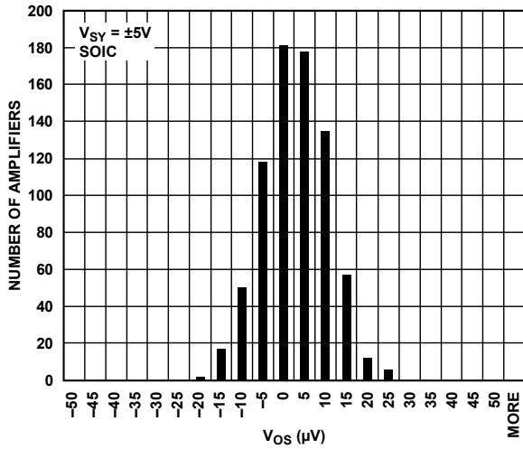
图10. 输入失调电压漂移( TCV_{OS} )分布, V_{SY} = \pm 5\text{V}
