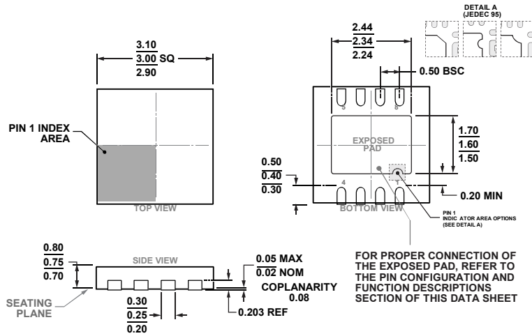
图67. 8引脚引线框芯片级封装[LFCSP]
