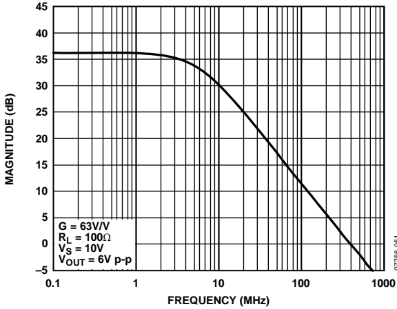
图52. 光电二极管前置放大器频率响应
