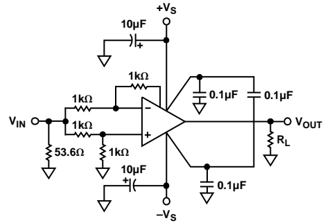
图40. 共模抑制
