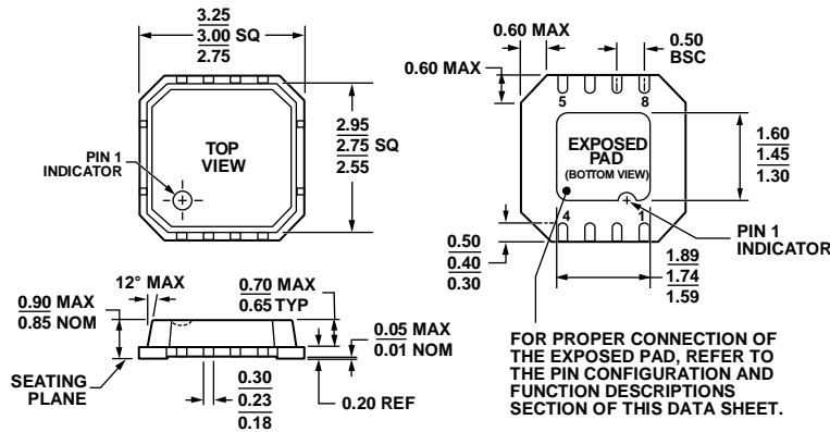
图58. 8引脚引脚架构芯片级封装[LFCSP_VD] 3 mm x 3 mm, 超薄体, 双列引脚(CP-8-2) 尺寸单位: mm
