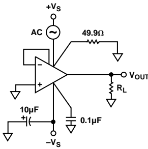
图36. 正电源抑制
