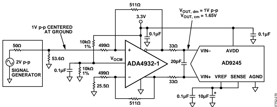
图66. ADA4932-1驱动AD9245 ADC，直流耦合输入和输出布局布线、接地和旁路
