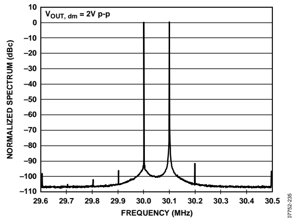
图35. 30 MHz交调失真
