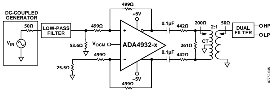
图54. 失真测量的测试电路
