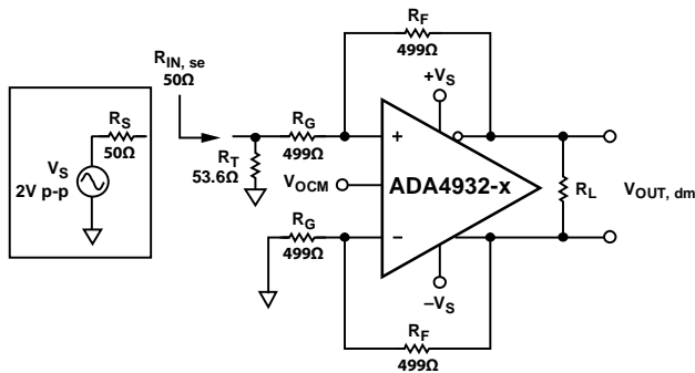
图60. 添加端接电阻 R_T
