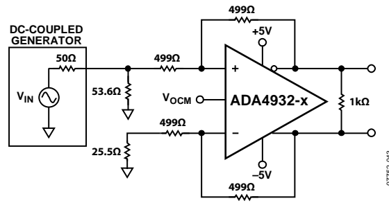
图52. 等效基本测试电路, G = 1
