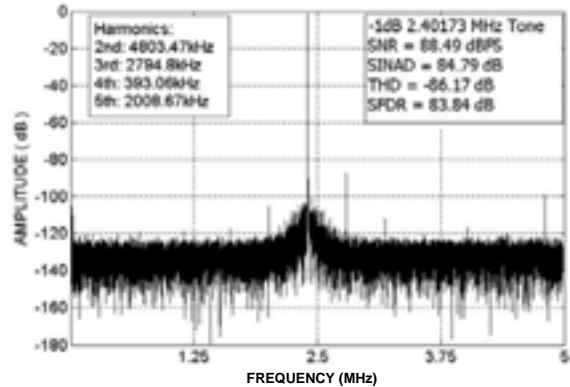
图64. AD7626输出，64,000点，FFT曲线-1 dBFS幅度，2.40173 MHz输入信号音，10.000 MSPS采样速率
