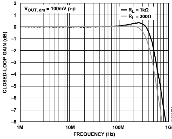
图14. 不同负载下的小信号频率响应
