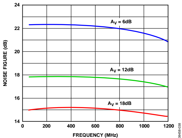
Figure 7. Noise Figure vs. Frequency at AV = 6 dB, AV = 12 dB, and AV = 18 dB
