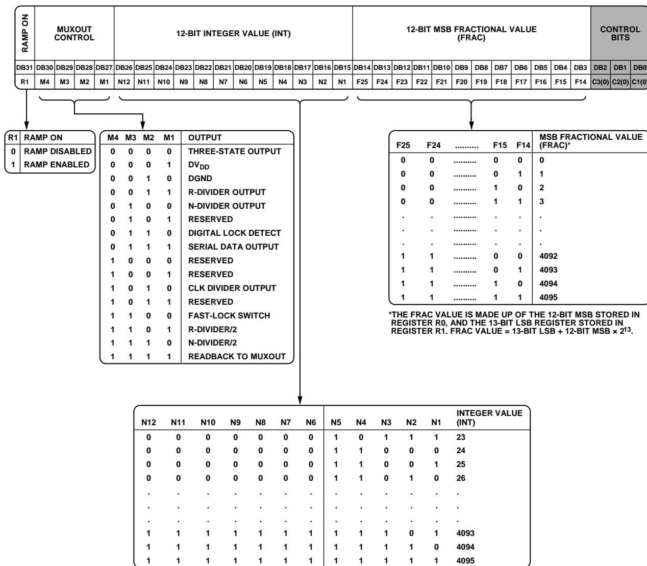
图23. FRAC/INT寄存器(R0)映射
