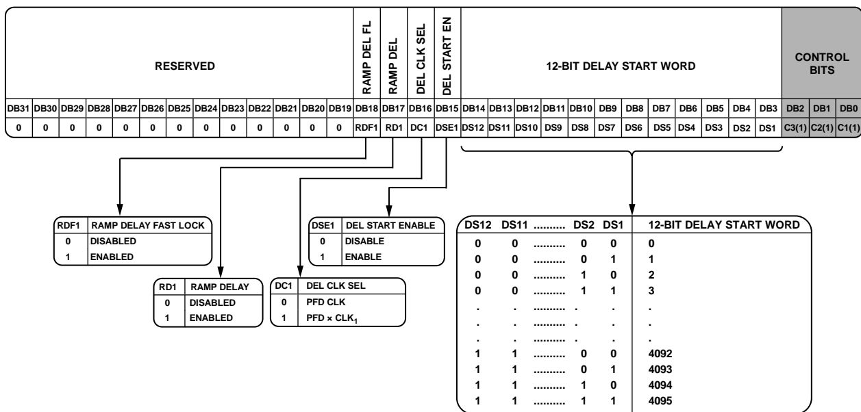
图30. 延迟寄存器(R7)映射
