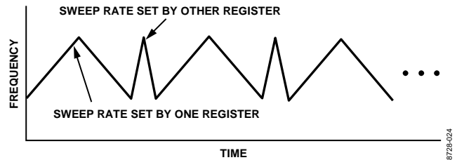
图36. 双扫描速率
