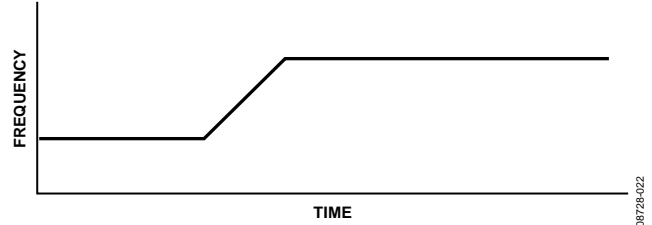
图31. 单一斜坡突发脉冲
