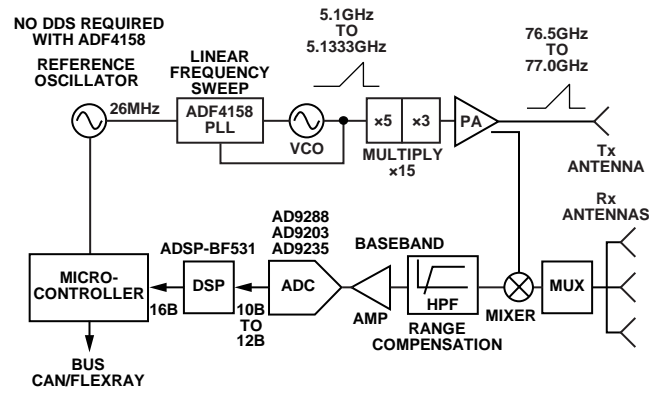
图47. 采用ADF4158的FMCW雷达
