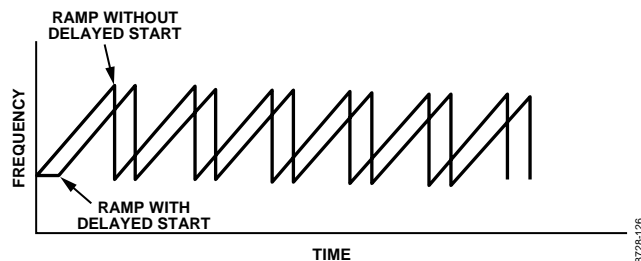
图38. 锯齿斜坡的延迟启动
