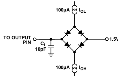
图4. MUXOUT时序的负载电路( C = 10 pF)
