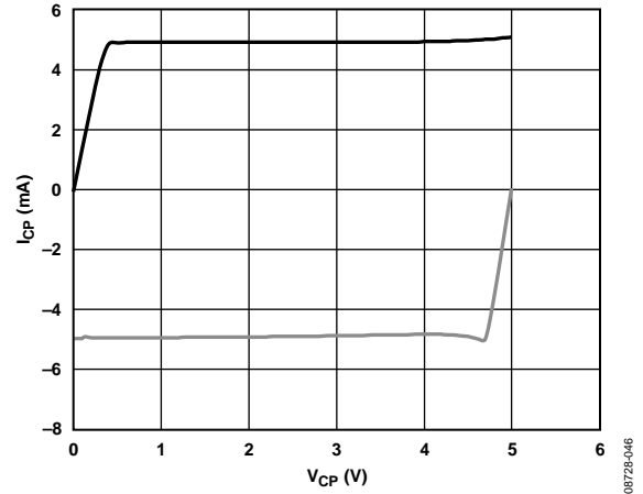
图15. 电荷泵输出特性
