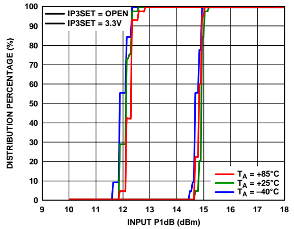
Figure 30. Input P1dB
