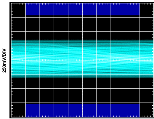
0.125UI/DIV AT 2.25Gbps
