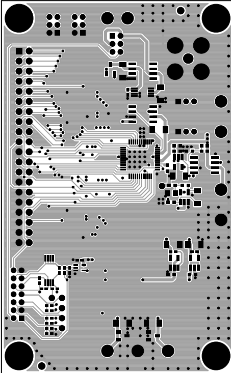
Layer 1-Top Layer
