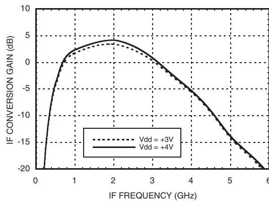
IF Bandwidth @ LO = -4 dBm
