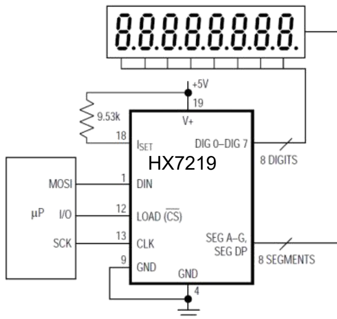
8-DIGIT \mu P DISPLAY
