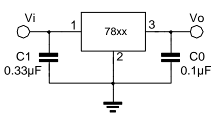
图1 测直流电参数电路图
