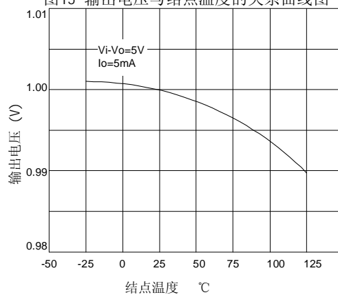
图15 输出电压与结点温度的关系曲线图
