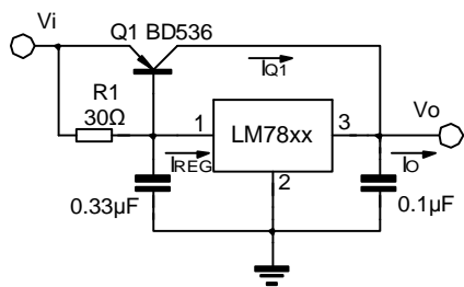
I_o = I_{REG} + (I_{REG} - V_{BEQ1} / R1) R1 = V_{BEQ1} / (I_{REG} - I_{Q1}) 图8 高电流电压稳压电路
