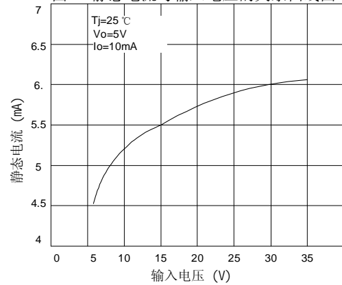
图17 静态电流与输入电压的关系曲线图
