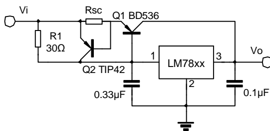
R_{sc} = V_{BEQ2} / I_{sc} 图9 高输出电流短路保护电路
