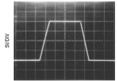
A_V = +1
