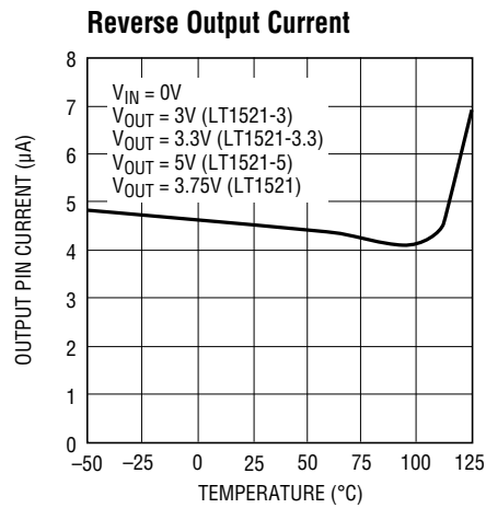
LT1521 • TPC29
