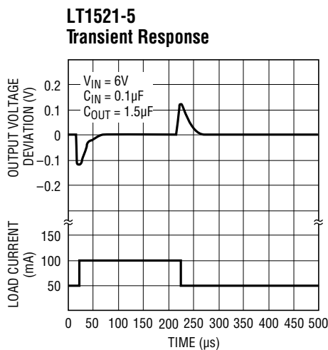
LT1521 • TPC33
