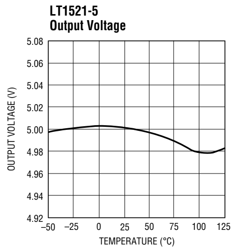
LT1521 • TPC06
