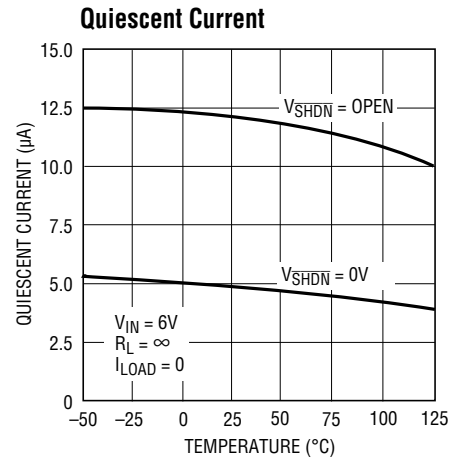
LT1521 • TPC03
