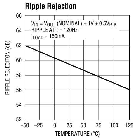
LT1521 • TPC30
