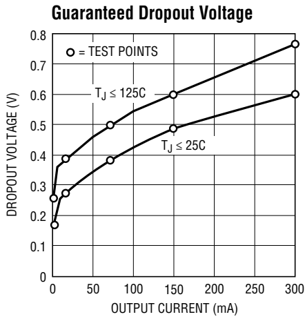
LT1521 • TPC01
