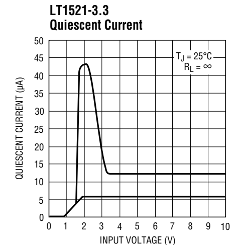
LT1521 • TPC09
