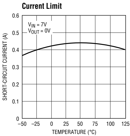
LT1521 • TPC28
