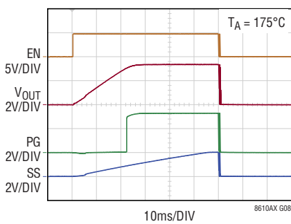
EN Cycling at 175°C
