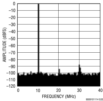
LTM9009-14: 8k Point FFT, f_{IN} = 70\text{MHz} , -1\text{dBFS} , 80\text{Mpsps}
