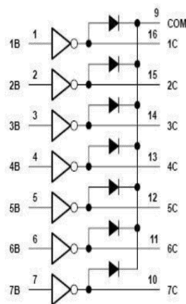
ULN2003 逻辑图
