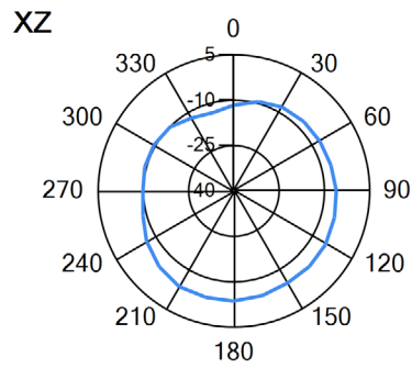
— 764MHz
