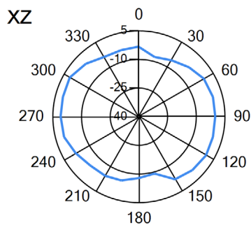
— 2.34GHz
