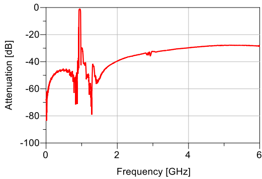
Attenuation
