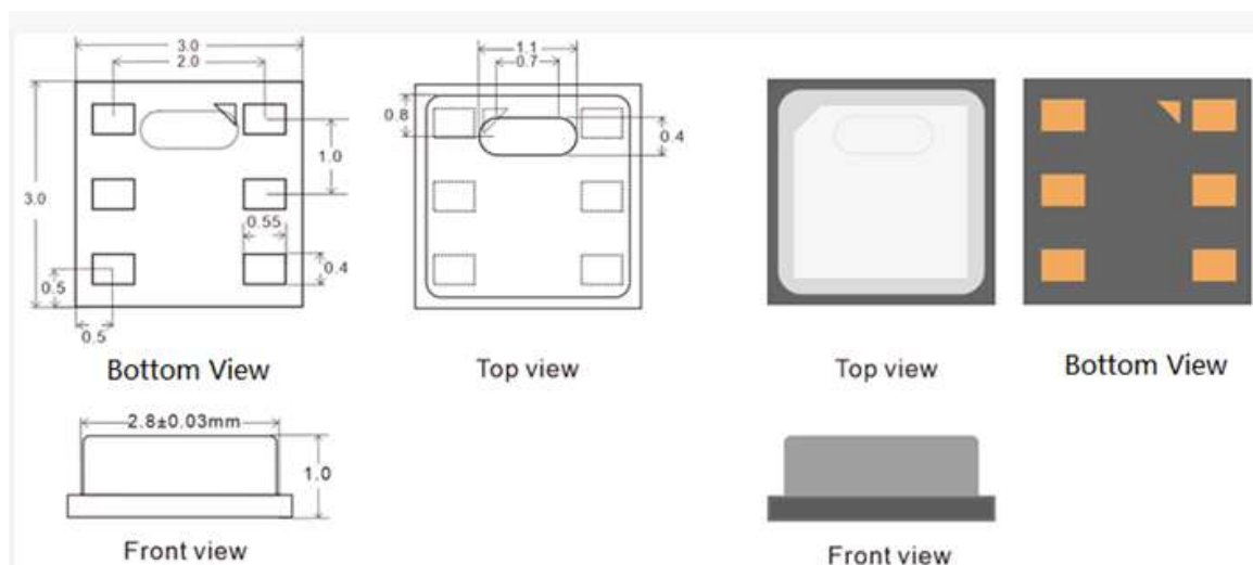
图 1: AHT20-F传感器封装图(单位: mm 公差: ±0.1mm)
