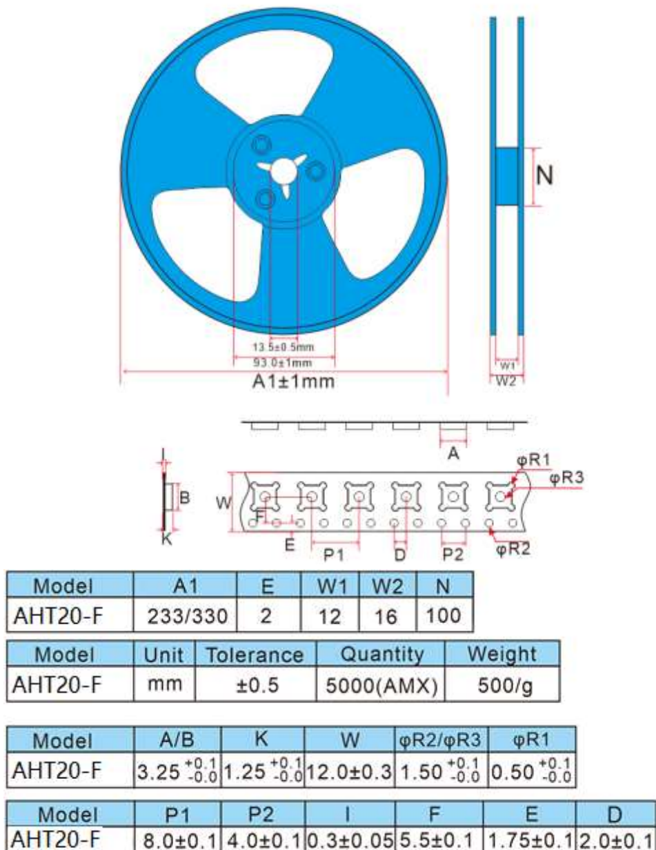
图21 包装卷带和传感器定位图
