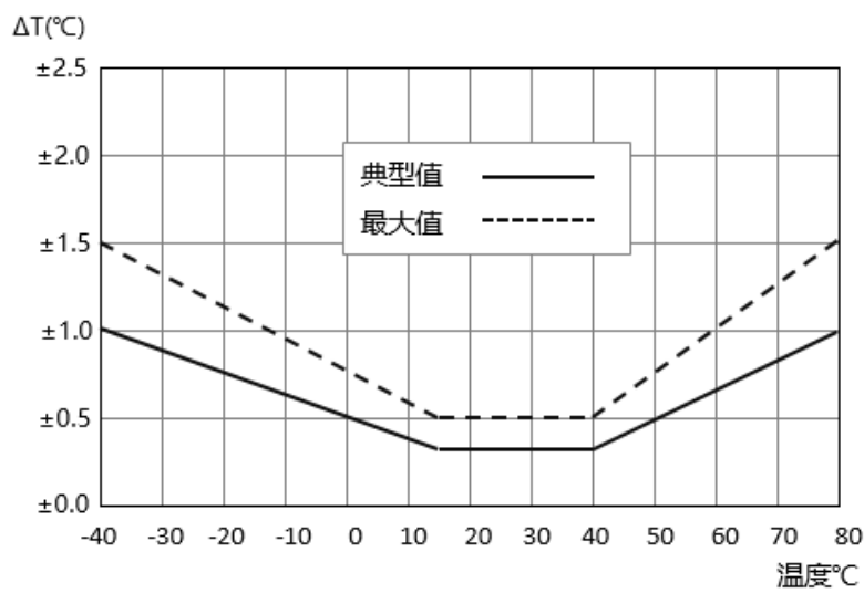
图3 温度典型误差和最大误差
