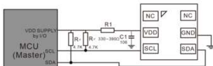
图15 典型应用电路。
