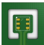
图10 AHT21 印刷电路板俯视图，图中加入铣削狭缝的设计，可以将热传递降低到最小。
