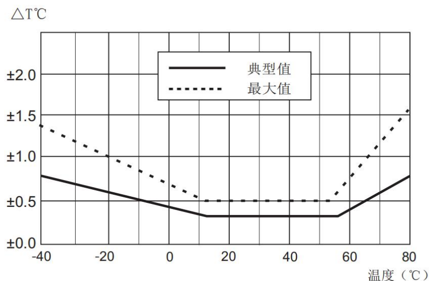
图3 温度典型误差和最大误差
