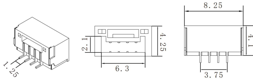
图13 AM2108 传感器连接器图标 (单位: mm不指定公差: 0.3mm)
