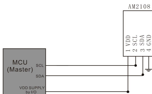
图8 典型的应用电路
