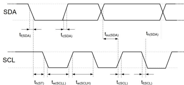
图9 数字输入/输出端的时序图、缩略语在表7中进行了解释。
