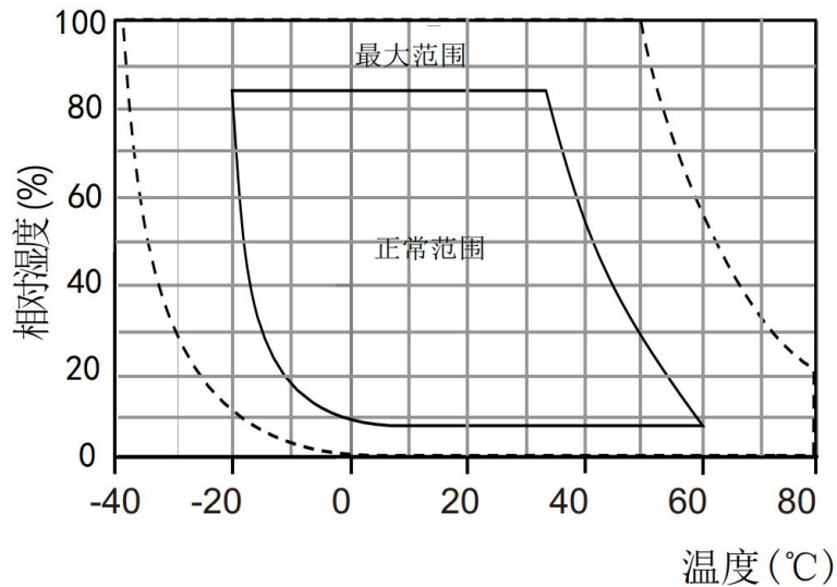
图4 工作条件
