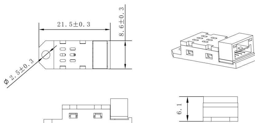
图12 AM2108 传感器封装图（单位：mm未标明公差：0.5mm）。
