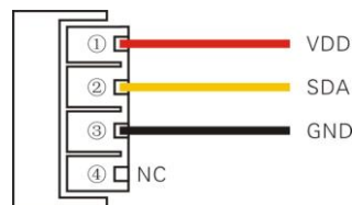
图 1：AM2301 引脚分配图
