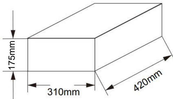
小纸箱尺寸图：公差±5mm
