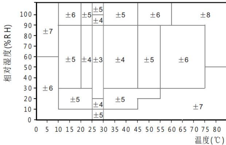
图5. 0~80℃范围内对应的湿度典型误差，单位：(%RH) 请注意：以上误差为以高精度露点仪做参考仪器测试的典型误差(不包括迟滞)。
