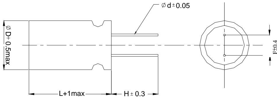
Fig. 2 Dimension
