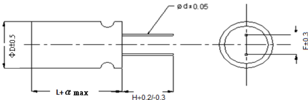
Fig. 2 Dimension
