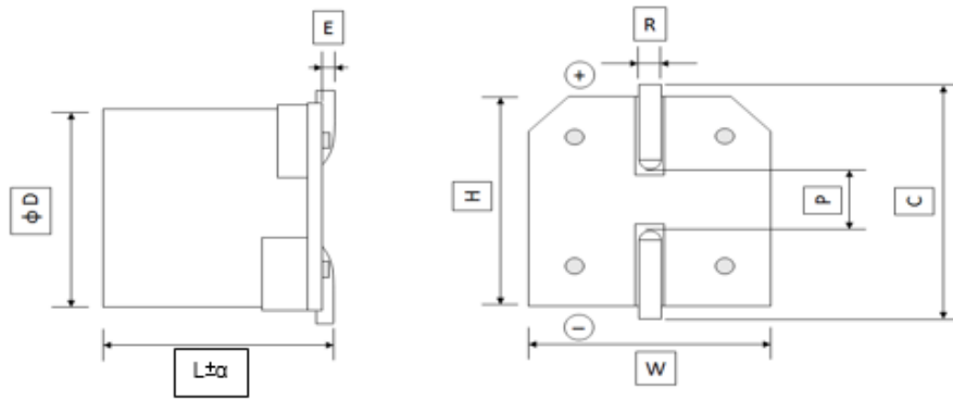
Fig. 2 Dimension
