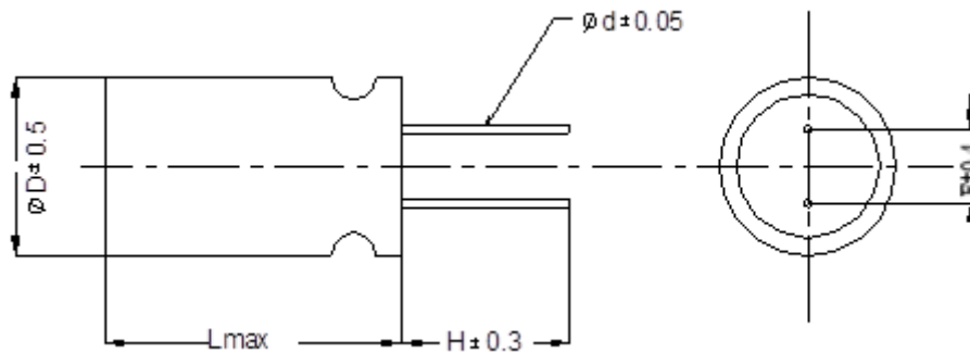
Fig. 2 Dimension
