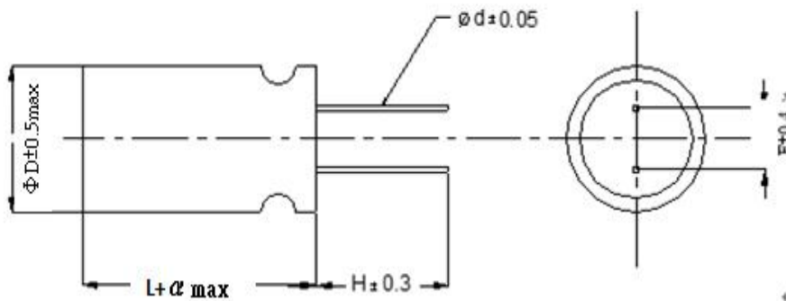
Fig. 2 Dimension
