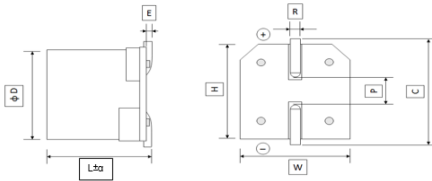
Fig. 2 Dimension
