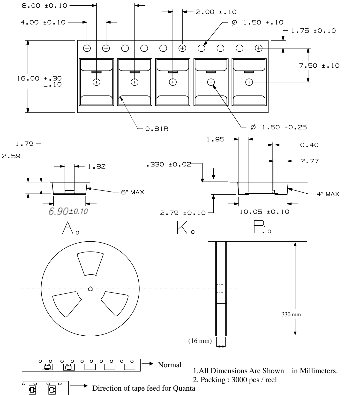
附圖一：Tape & Reel Information : TO-252
