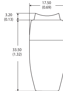
AE Rocker
