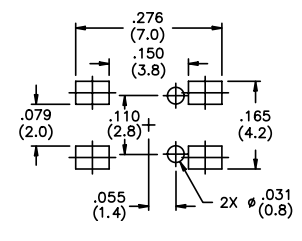
MJTP1140
