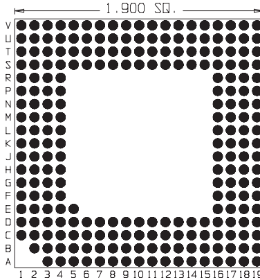
238 Pins Footprint 19004
