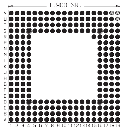
238 Pins Footprint 19007 - ZIF
