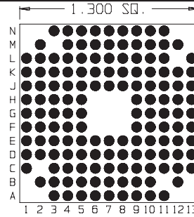
144 Pins Footprint 13095
