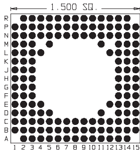
149 Pins Footprint 15019
